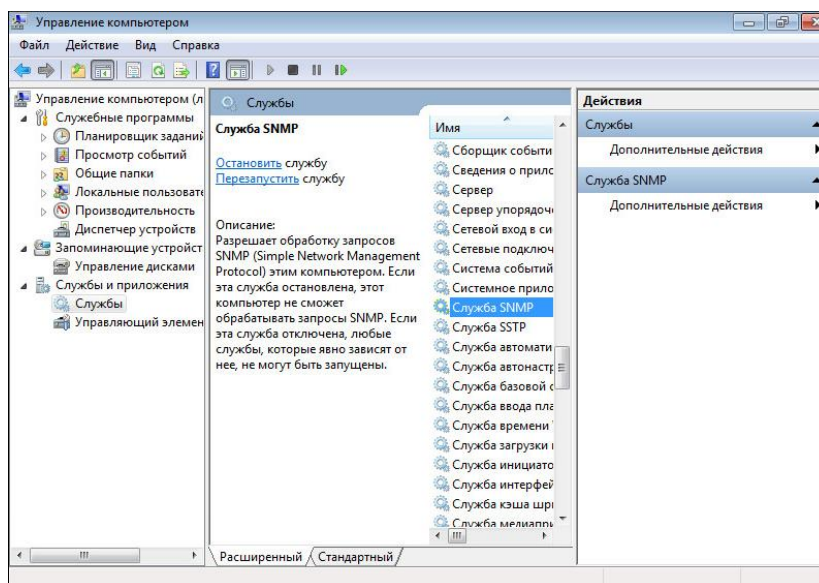
Рисунок 20 – Службы SNMP
