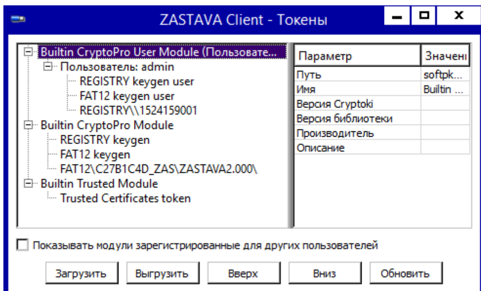
Рисунок 57 – Окно «Токены»
