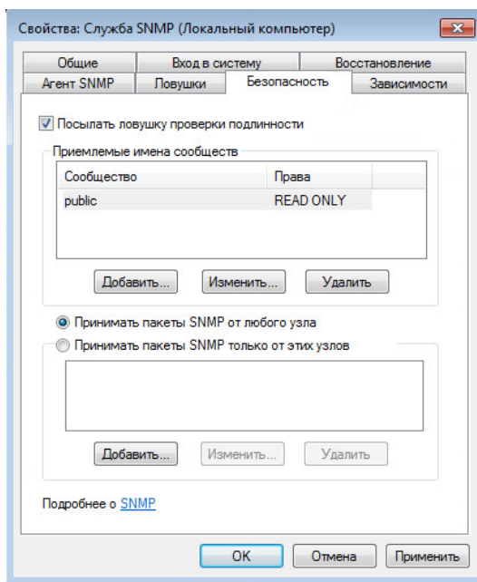
Рисунок 21 – Службы SNMP
