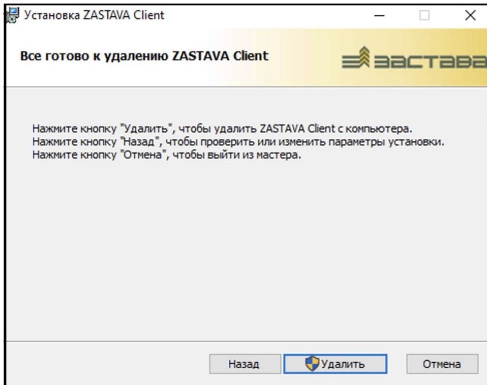
Рисунок 13 – Подтверждение удаления
