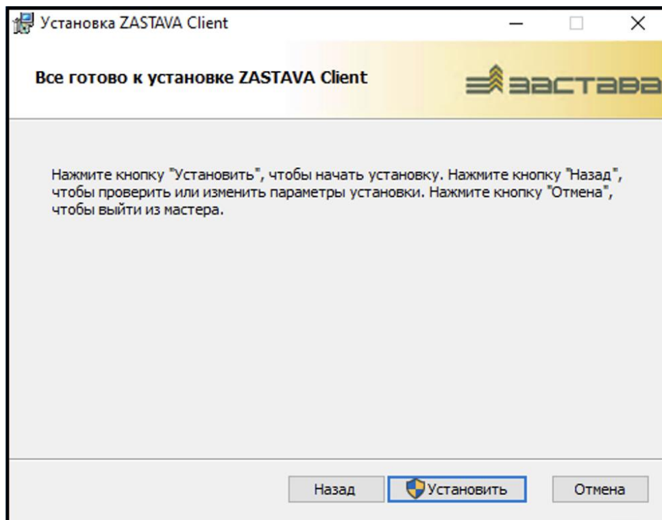
Рисунок 6 – Подтверждение установки
