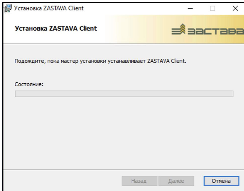
Рисунок 7 – Окно установки
