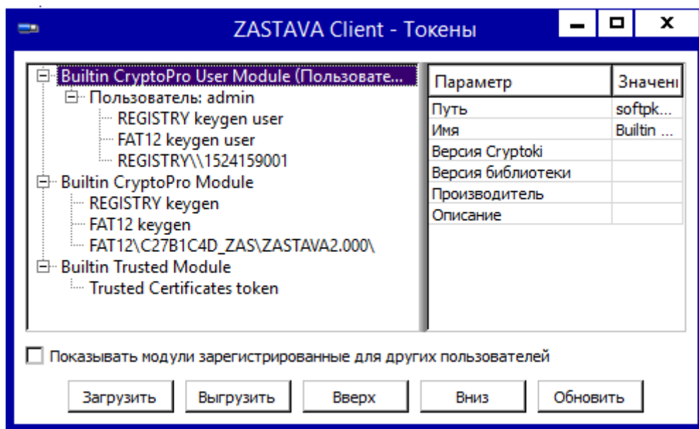
Рисунок 59 – Окно «Токены»
